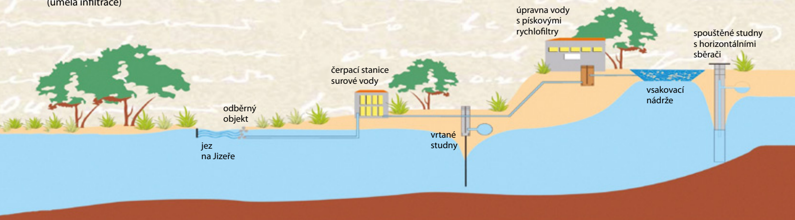
Schéma úpravy vody (umělá infiltrace)
